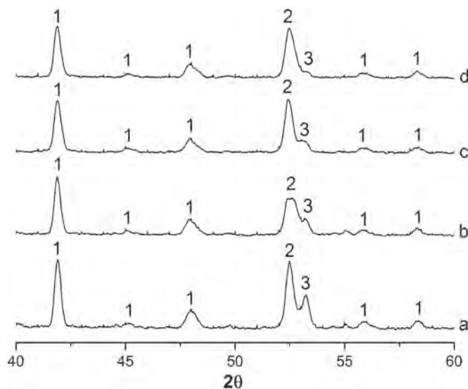
Рис. 1. Фрагменты рентгенограмм продуктов азотирования ФСА, 10% маршаллита и предварительно азотированного порошка (добавка предварительно азотированного: а – 10%, б – 20%, в – 28,5%, д – 30%; 1 – \beta -SiAlON, 2 – \alpha -Fe, 3 – Fe_xSi_y )
