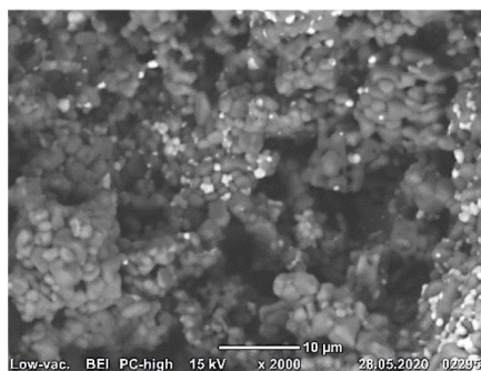
Рис. 2. Скол пористой алюмоциркониевой керамики
