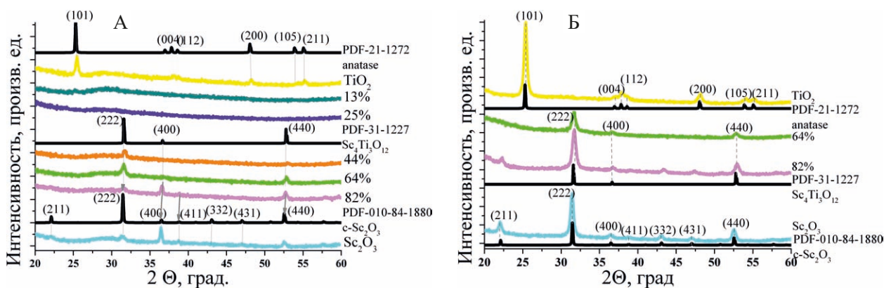
Рис. 1. Дифрактограммы плёнок \text{Sc}_x\text{Ti}_{1-x}\text{O}_y , полученных на различных подложках: А – планарном кремнии, Б – чёрном кремнии
