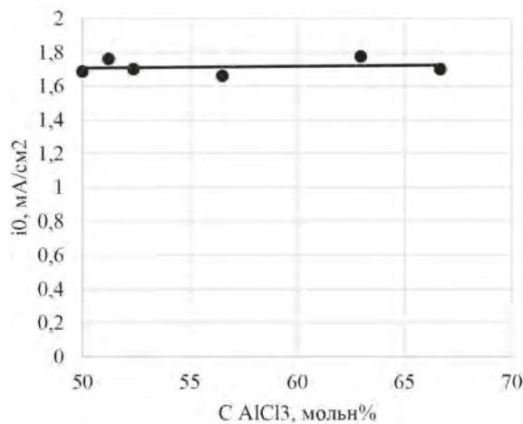
Рис. 1. Зависимость i_0 от молярной доли AlCl_3 на границе Al|AlCl_3-[EMIm]Cl
