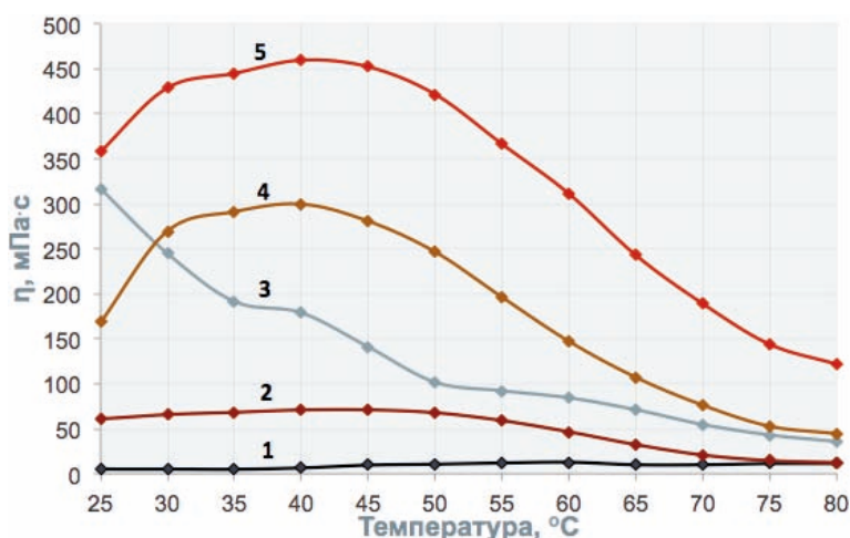
Рис. 1. Зависимость эффективной вязкости исследуемых систем от температуры при 100 \text{ с}^{-1} 1 – 0,2% МЦ; 2 – 2% ВУПАВ; 3 – 2% ВУПАВ+0,5% \text{AlCl}_3 ; 4 – 2% ВУПАВ+0,2% МЦ; 5 – 2% ВУПАВ+0,5% \text{AlCl}_3 +0,2% МЦ. Вода остальное
