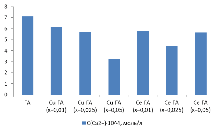
Рис. 1. Результаты растворимости образцов СиГА и СеГА в 0,9% (масс.) растворе NaCl
