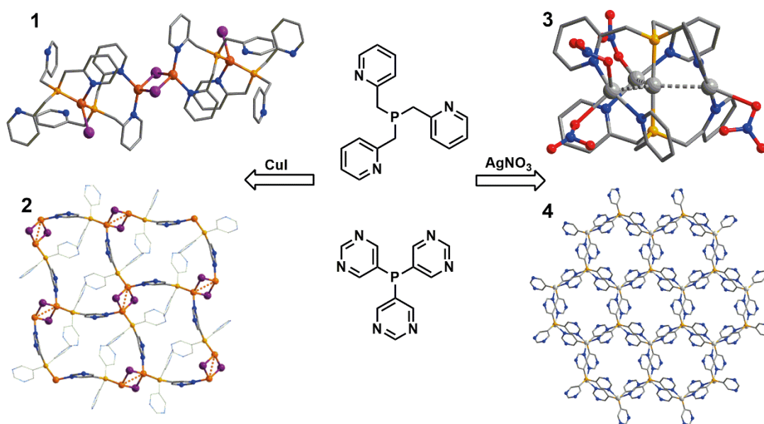
Схема 1. Молекулярные комплексы с AgNO_3 и CuI на основе трис(2-пиколил)фосфина и координационные полимеры на основе трис(5-пиримидил)фосфина
