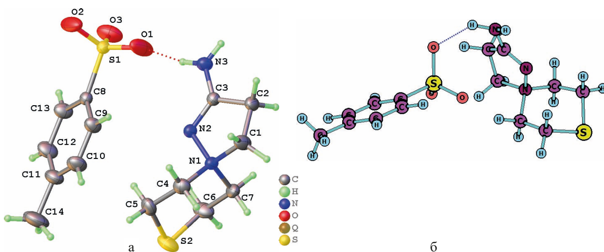
Рис. 1. (а) Данные PCA кристаллов продукта 8 . (б) Геометрия молекулы продукта 8 , рассчитанная методом ab initio HF/3-21G
