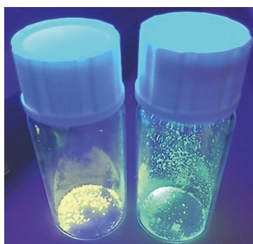
Рис. 2. (а) Фотолуминесценция ариновых комплексов Cu (I): слева – комплекс с трис(4-метоксифенил)арсином, справа – с трис(4-метилфенил)арсином. (б) Спектр эмиссии представлен для комплекса с трис(4-метоксифенил)арсином
