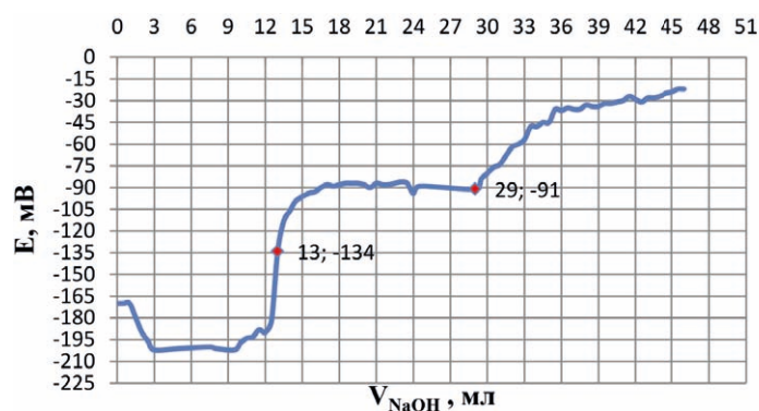
Рис. 1. Кривая титрования H_3PO_4
