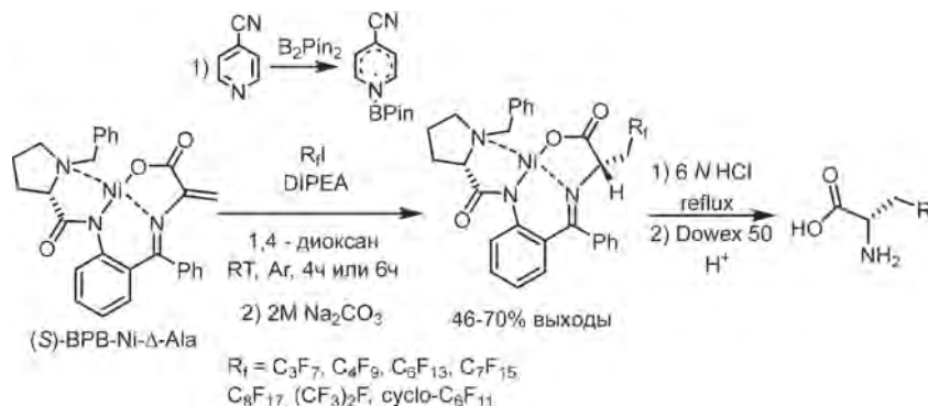
Схема 2. Радикальная реакция перфторалкилирования
