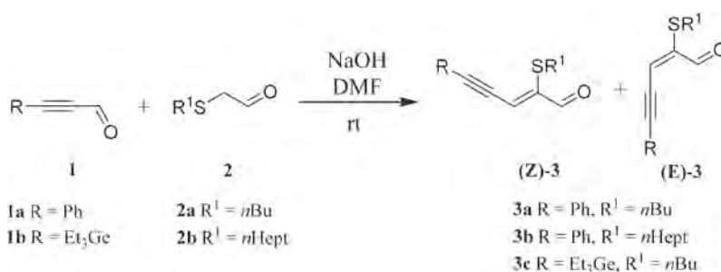
Схема 1. Синтез 2-тиозамещенных 2-ен-4-иналей
