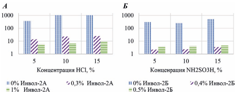
Рис. 1. Зависимость плотности тока коррозии в присутствии различных концентраций ингибитора Ивол-2А от концентрации соляной кислоты (А) и Ивол-2Б от концентрации сульфаминовой кислоты (Б), t = 21 \pm 2^\circ\text{C} , \tau = 24 часа
