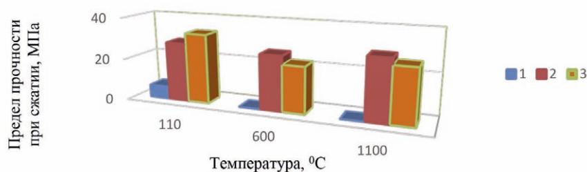
Рис. 1. Изменение предела прочности при сжатии исследованных составов с добавками терморасширяющегося графита (1), древесного угля (2) и углеродистого волокна (3)
