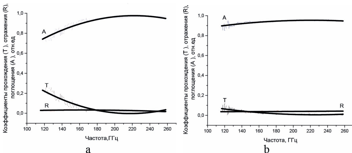
Рис. 2. Зависимость коэффициентов поглощения (А), отражения (R) и прохождения (Т) ЭМИ от частоты для пористого стеклокомпозита со средним размером пор на поверхности: а – 1,2 мм; б – 3,1 мм
