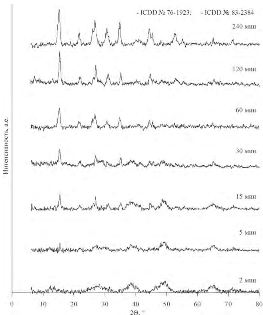
Рис. 1. Дифрактограммы продуктов реакции при различной продолжительности синтеза
