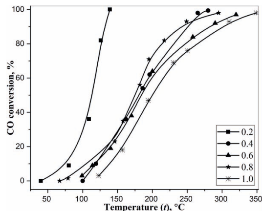
Рис. 1. Каталитическая активность полученных наноконпозитов
