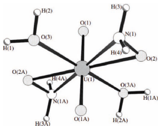
Рис. 1. Структура комплекса [UO_2(NH_2O)_2 \cdot (H_2O)_2]
