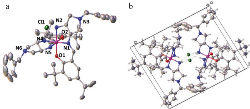
Рис. 2. Структуры комплексов 2 согласно данным РСА
