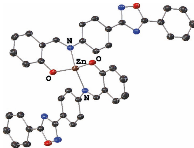
Рис. 2. Строение комплекса Zn(L_2)_2
