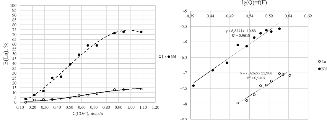
Рис. 1. Изотермы растворения лантана и неодима (III)
