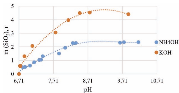
Рис. 1. Зависимость массы \text{SiO}_2 от pH осаждения
