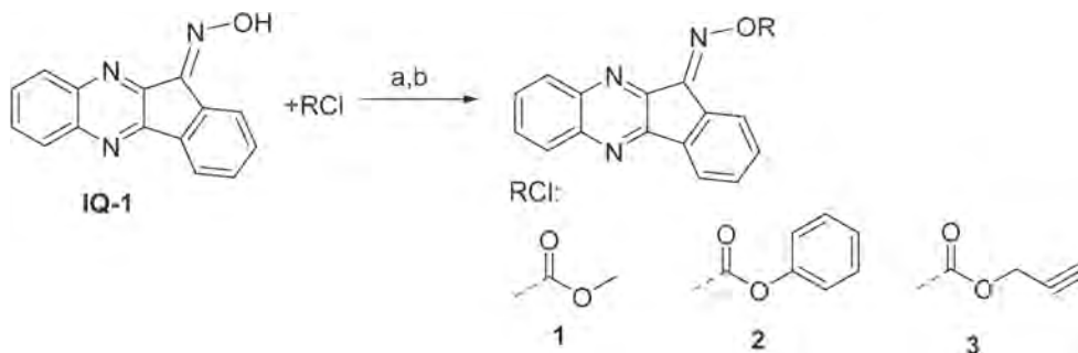
Схема 1. Условия реакций: a ) пиридин, 0 °С (Соединение 1 : 5 мин., выход 51%; соединение 2 : 30 мин., выход 86%, соединение 3 : 5 мин., выход 57%); b ) KOH-DMSO (Соединение 1 : 30 мин., выход 45%; соединение 2 : 30 мин., выход 68%; соединение 3 : 30 мин., выход 73%)
