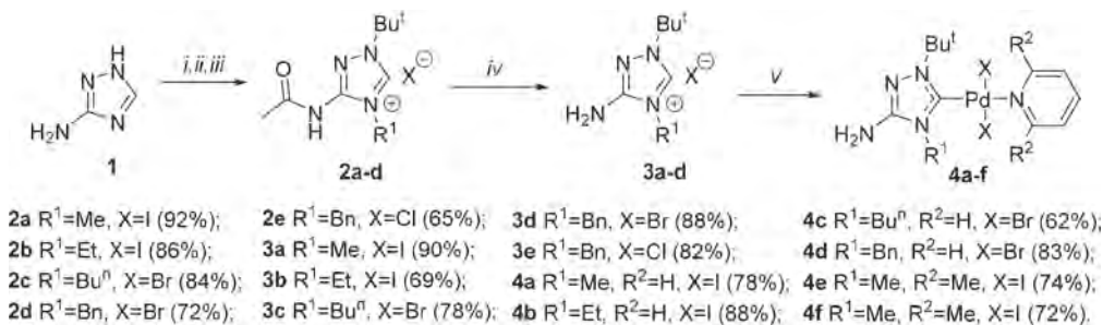
Схема 1. Синтез комплексов Pd–ННС со свободной аминогруппой
