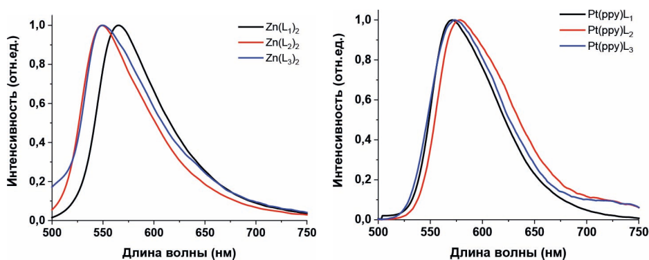
Рис. 3. Спектры фотолуминесценции оксадиазолсодержащих комплексов цинка и платины в твердом состоянии, \lambda_{ex} = 440 нм
