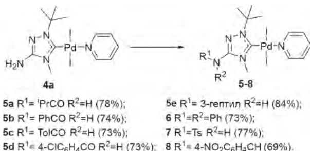
Схема 2. Постмодификация комплексов Pd–ННС со свободной аминогруппой
